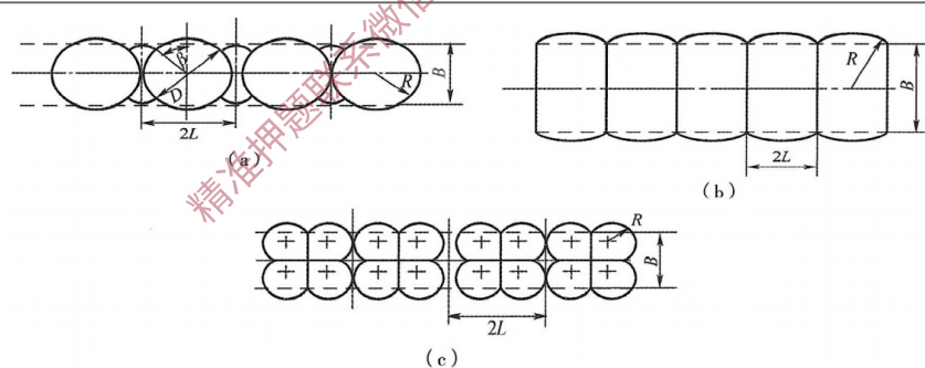
图 2.2-3 钢板桩格形围堰平面形式 (a) 圆筒形格体；(b) 扇形格体；(c) 花瓣形格体
